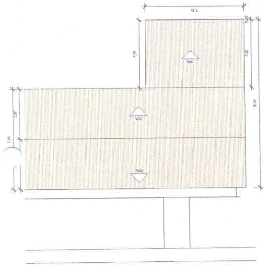
2 Estrutura do Telhado 1:100
