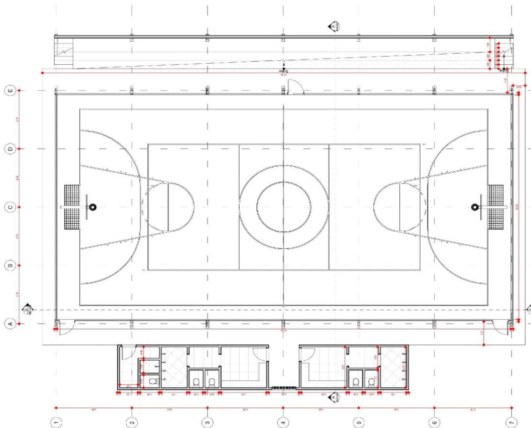
1 - PLANTA BAIXA - QUADRA POLIESPORTIVA COBERTA
