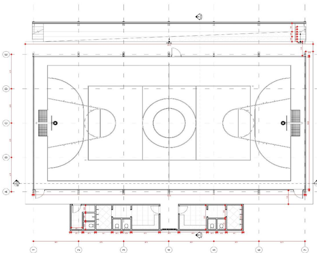
1 - PLANTA BAIXA - QUADRA POLIESPORTIVA COBERTA
