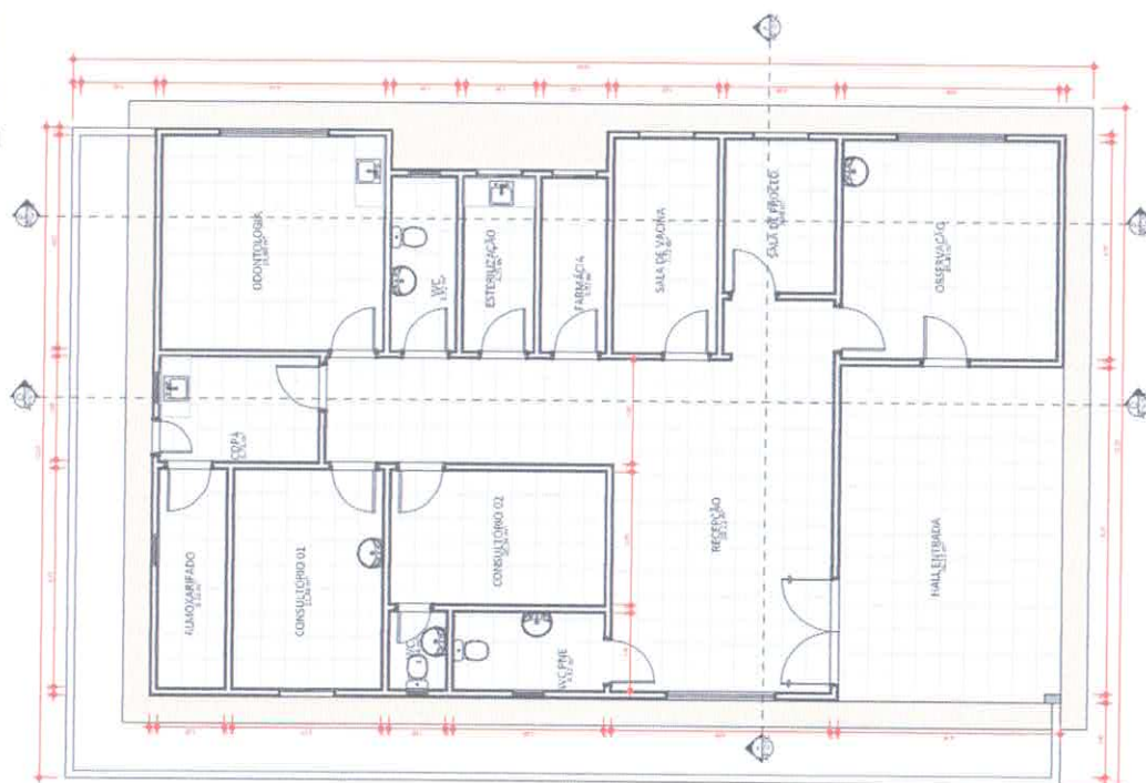
00.01, Planta Reforma
