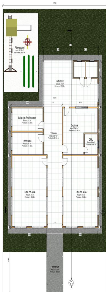
01 Planta Baixa Executiva Escala: 1:75
