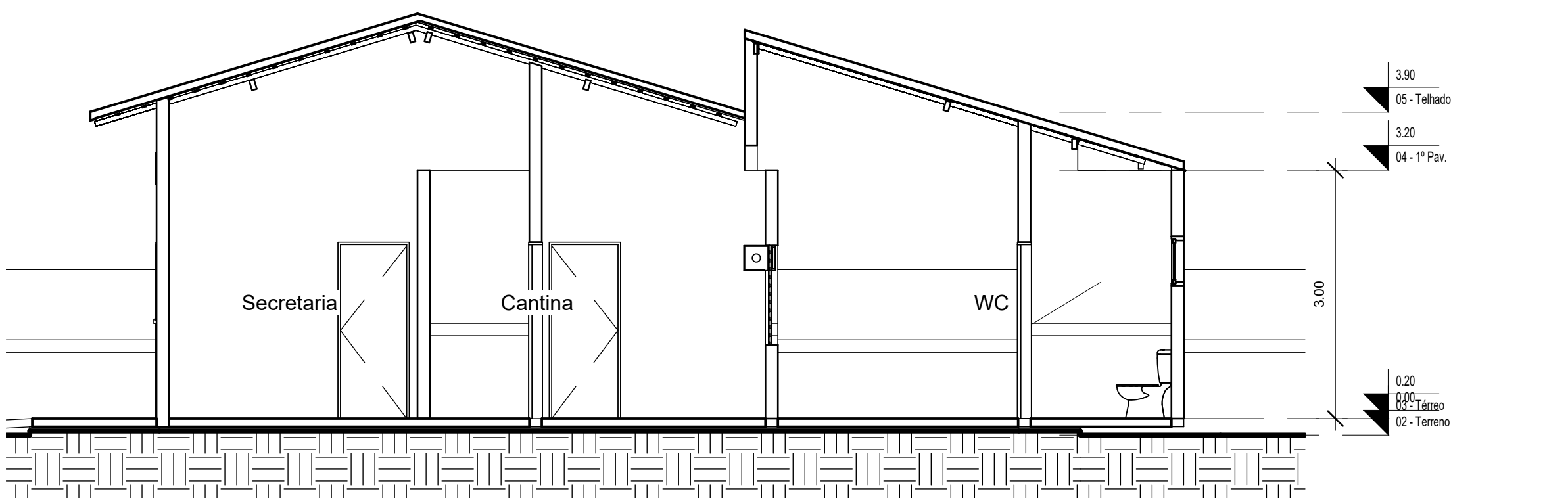
3 Corte AA 1 : 60
