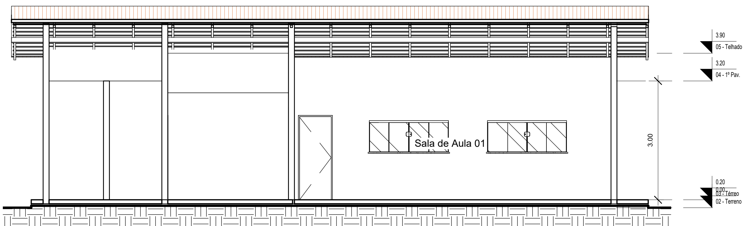
4 Corte BB 1 : 60
