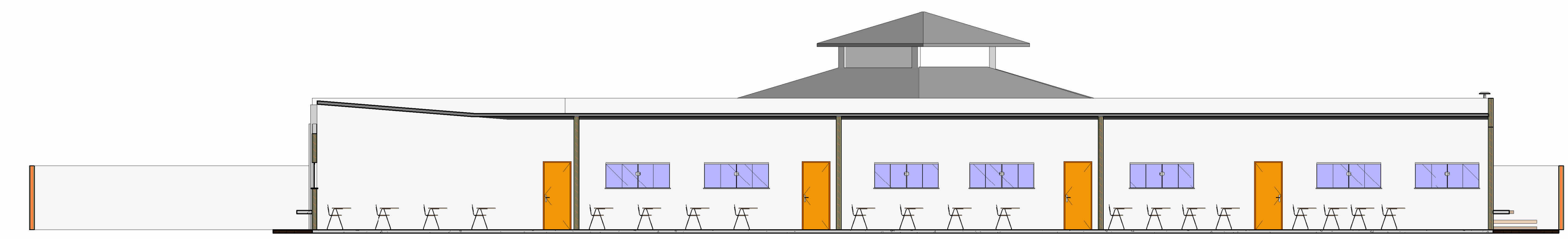
4 Vista Lateral Esquerda 1 : 100
