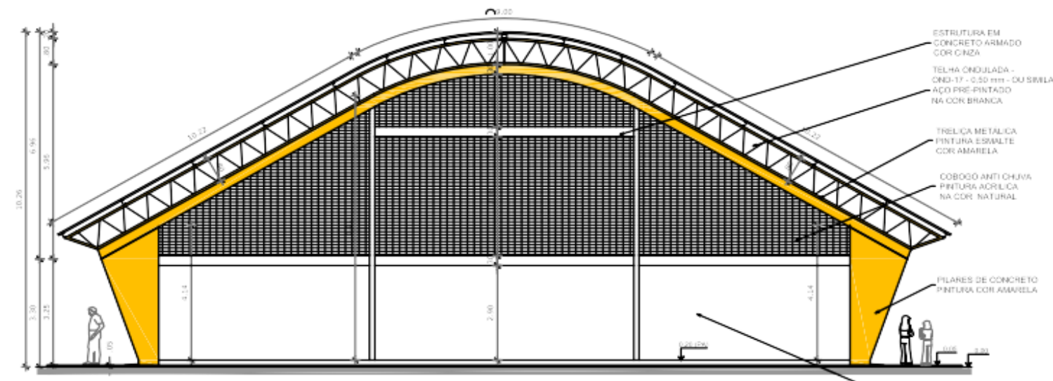
FACHADA 04 ESCALA 1:100
