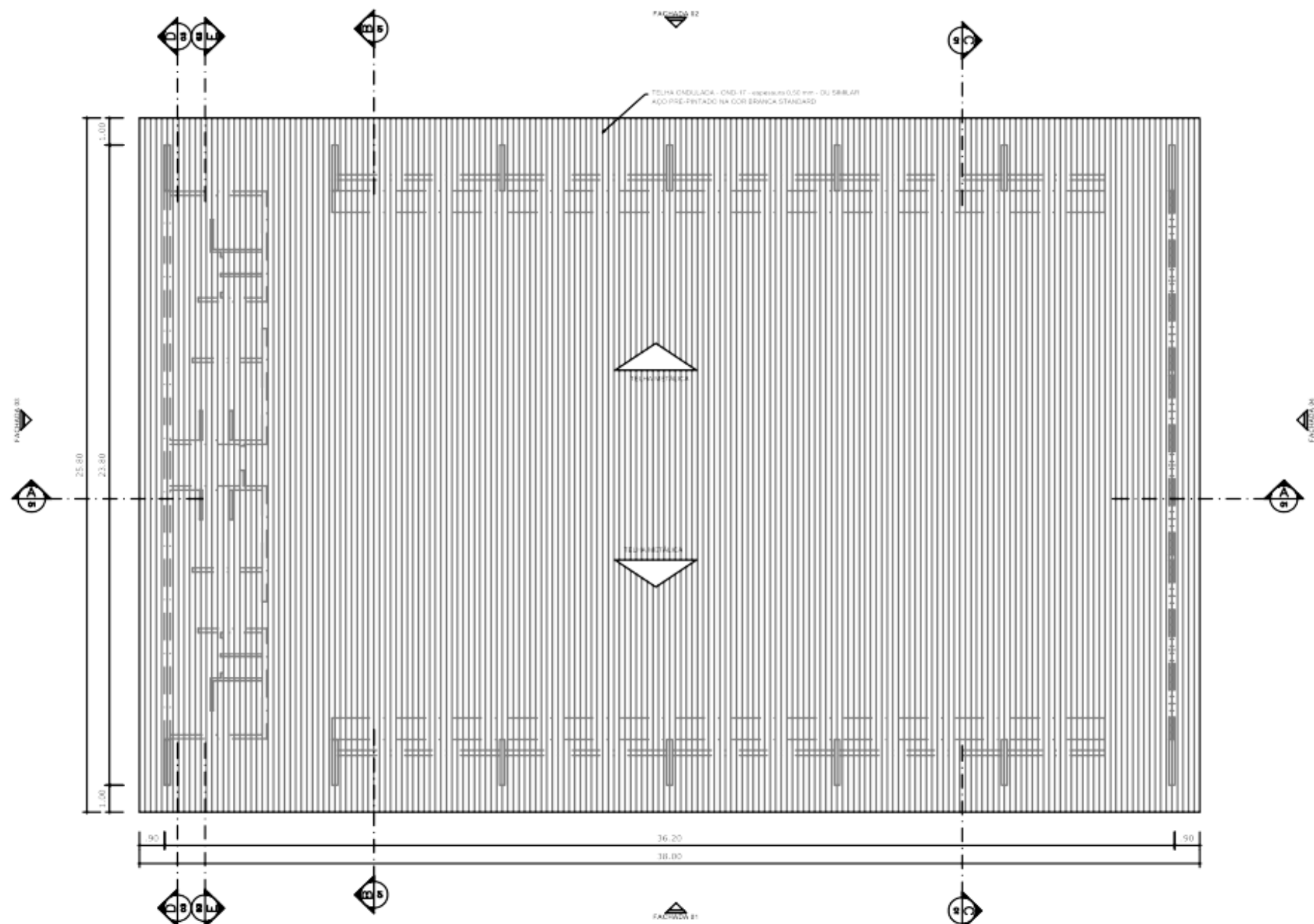
PLANTA DE COBERTURA ESCALA 1:125
