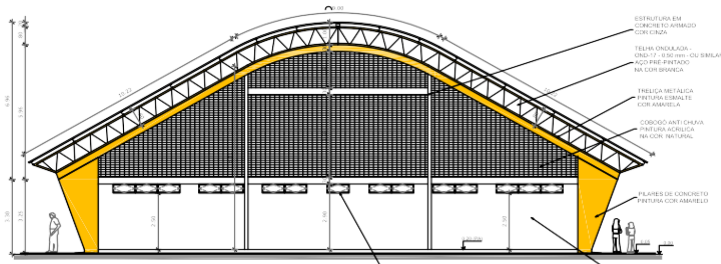
FACHADA 03 ESCALA 1:100
