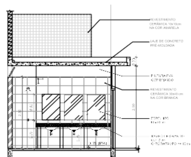
VESTIÁRIO: VISTA A
