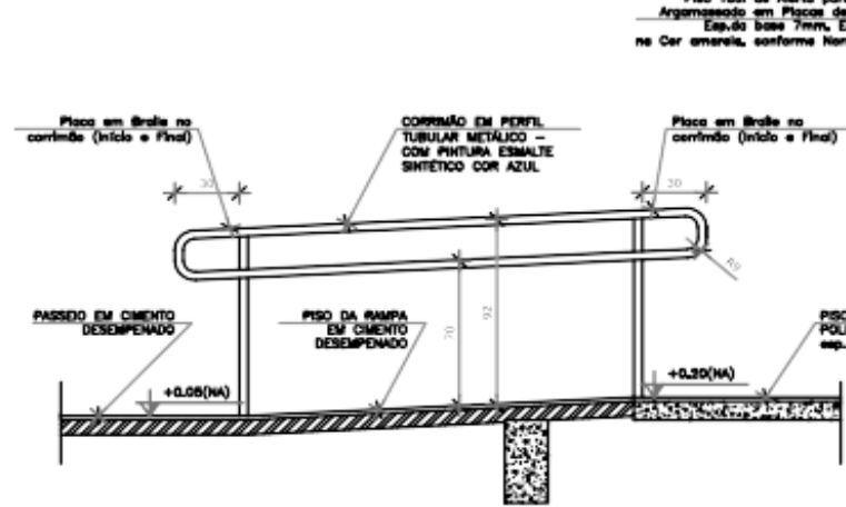
DETALHE 1 Escala: 1/5
