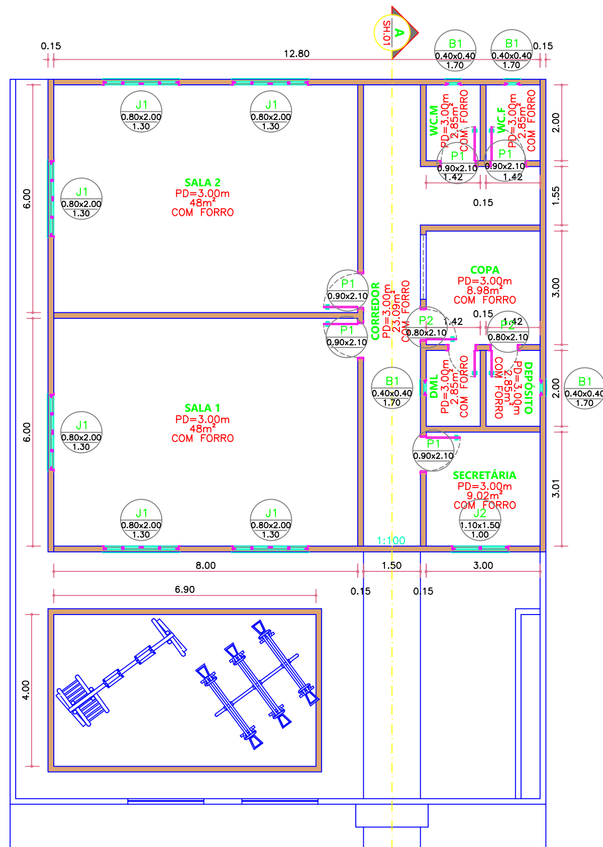
PLANTA BAIXA ESC. 1:100
