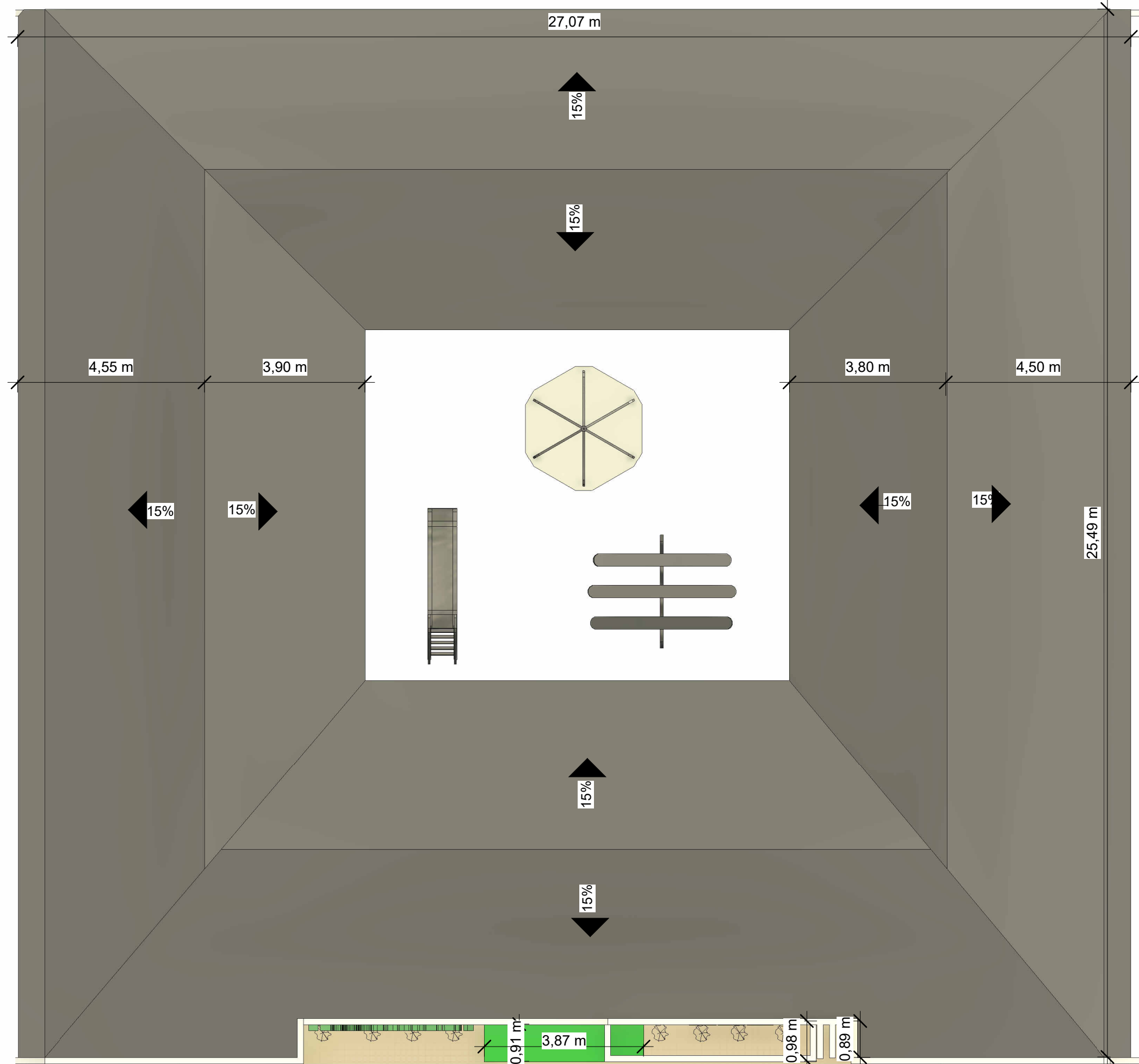
1 2.COBERTURA 1 : 100
