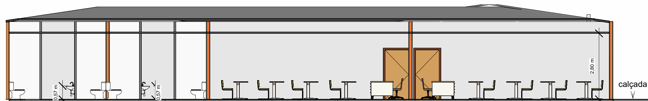
4 Corte B 1 : 100
