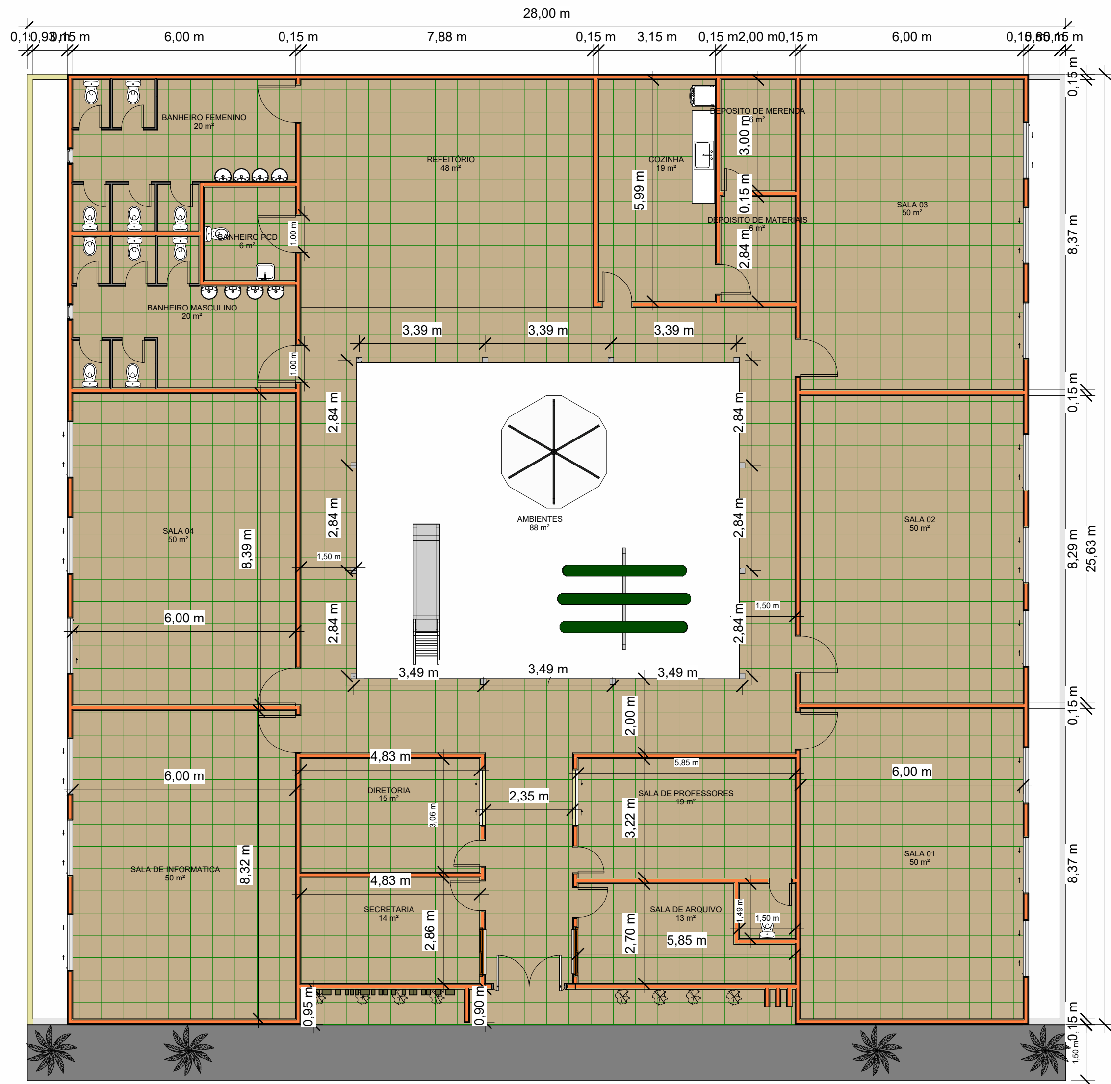
3 1. PLANTA BAIXA 1 : 100
