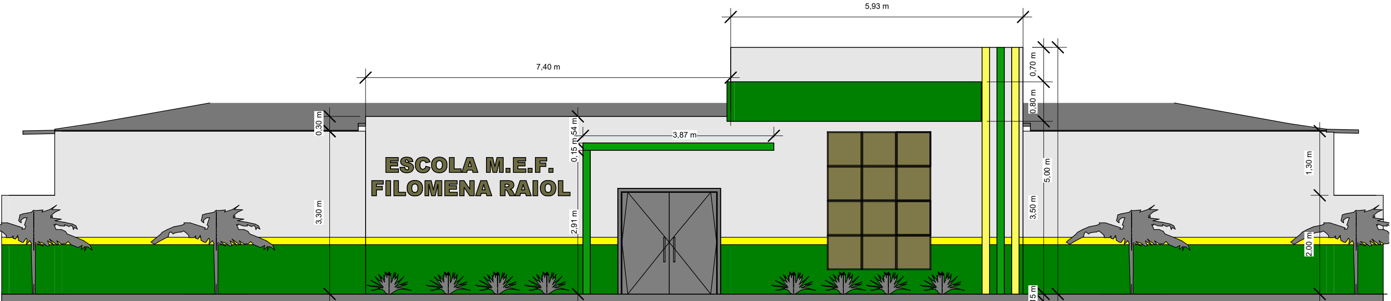
4 Corte Frontal 1 : 75
