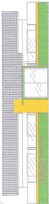
VISTA FRONTAL ESCALA 1/25
