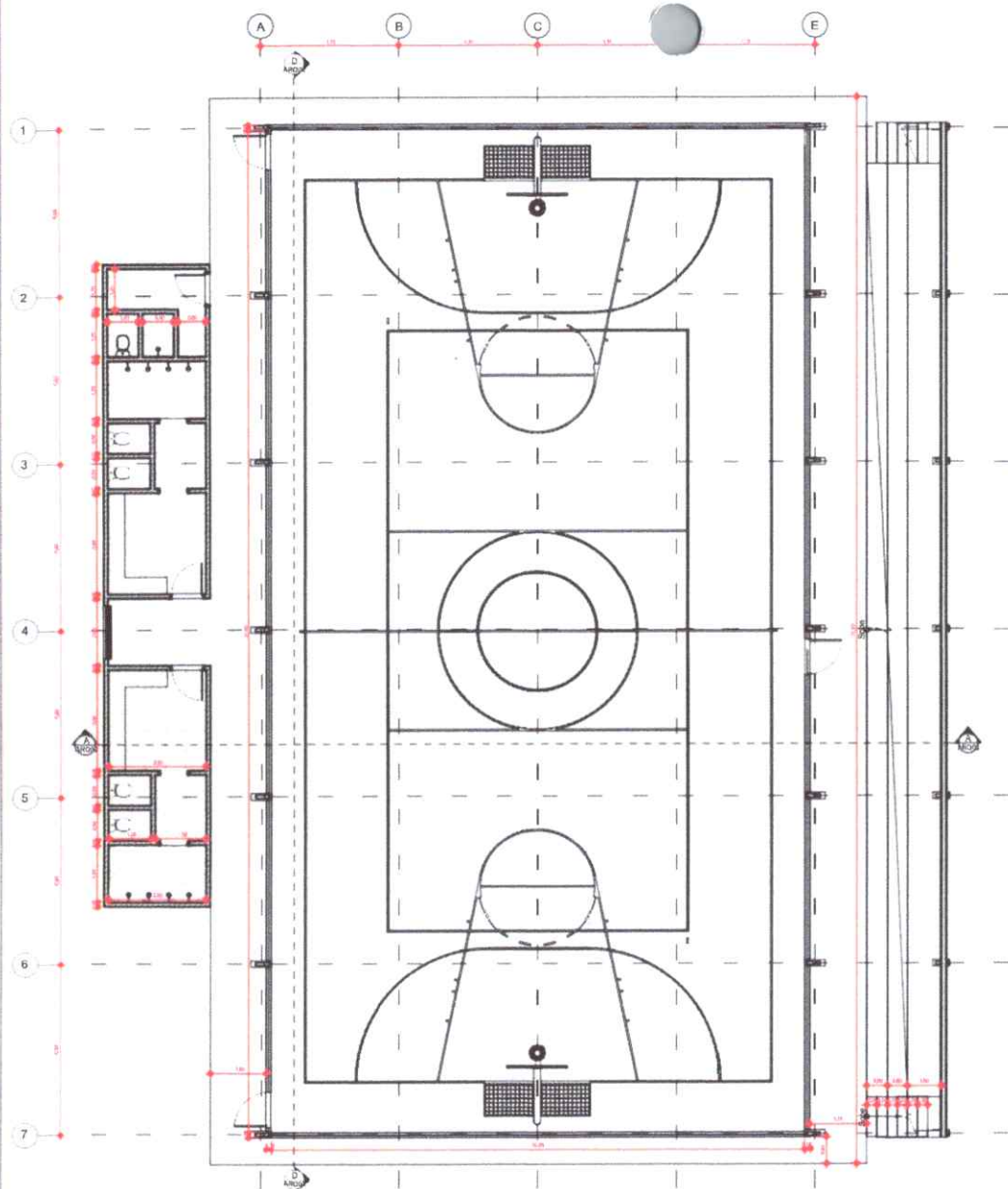
1 - PLANTA BAIXA - QUADRA POLIESPORTIVA COBERTA
