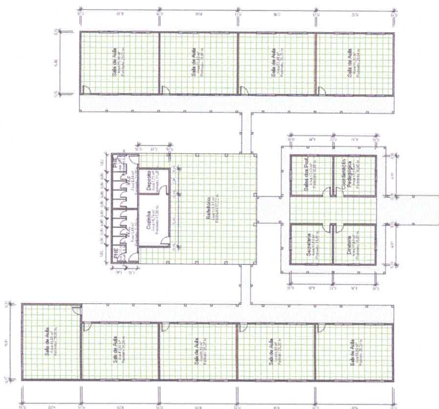
1 Planta Baixa Executiva 1-125
