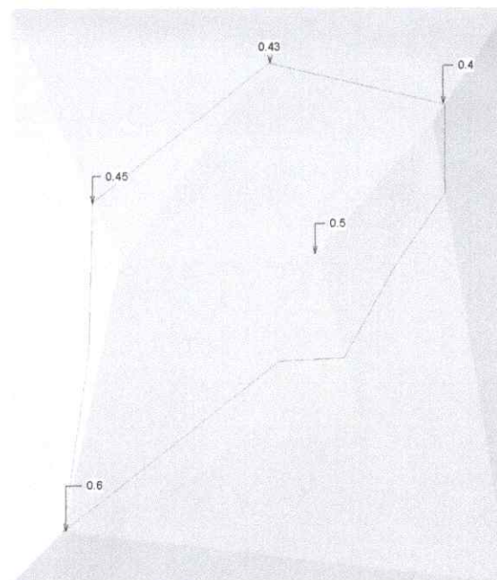
2 PLANIALTIMETRIA 1 : 100
