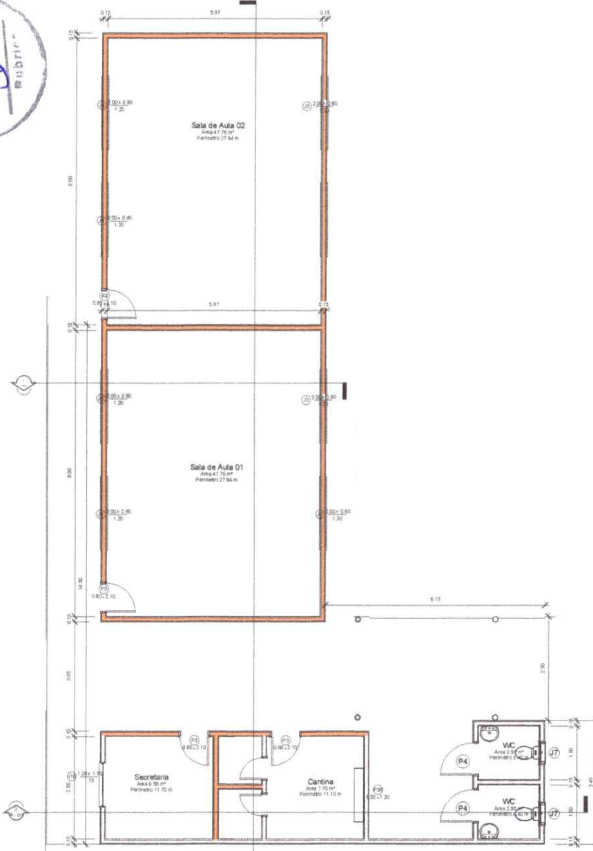
1 Planta Baixa Executiva 1 : 50
