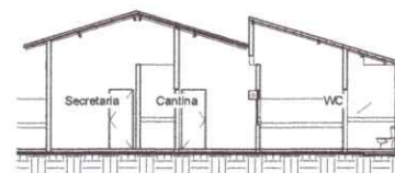
3 Corte AA 1 : 100
