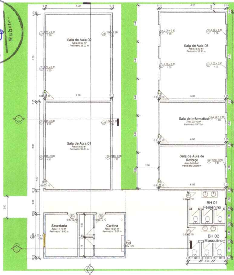
1 Planta Baixa Executiva 1:75
