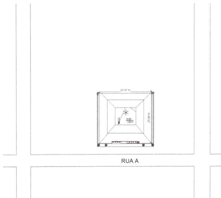
2 SITUAÇÃO 1 : 400
