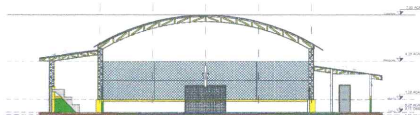
Elevação 1 - c
