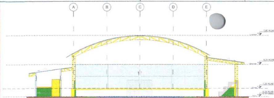
Corte A-A
