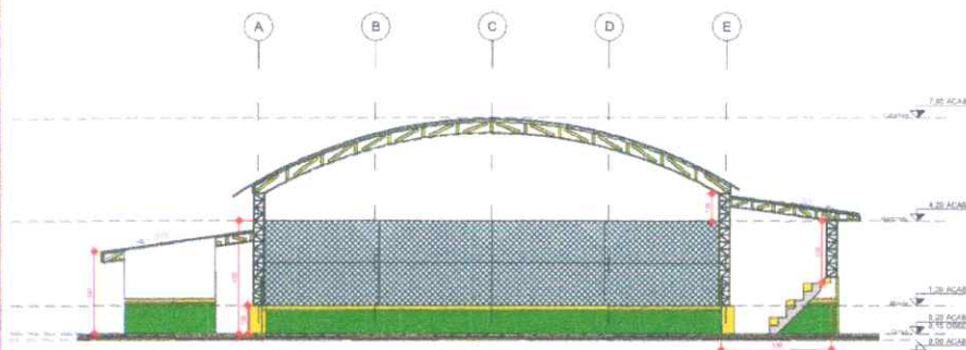
Corte A-A
