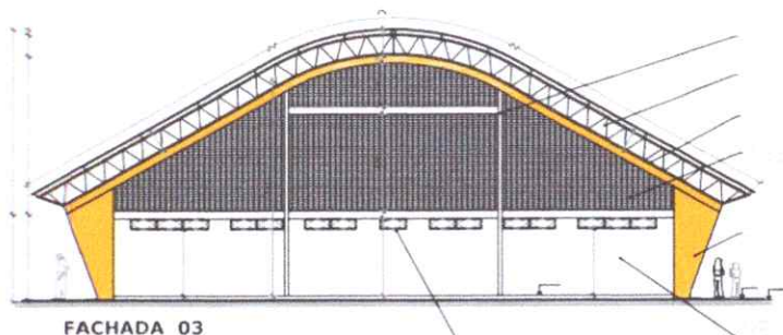
FACHADA 03
