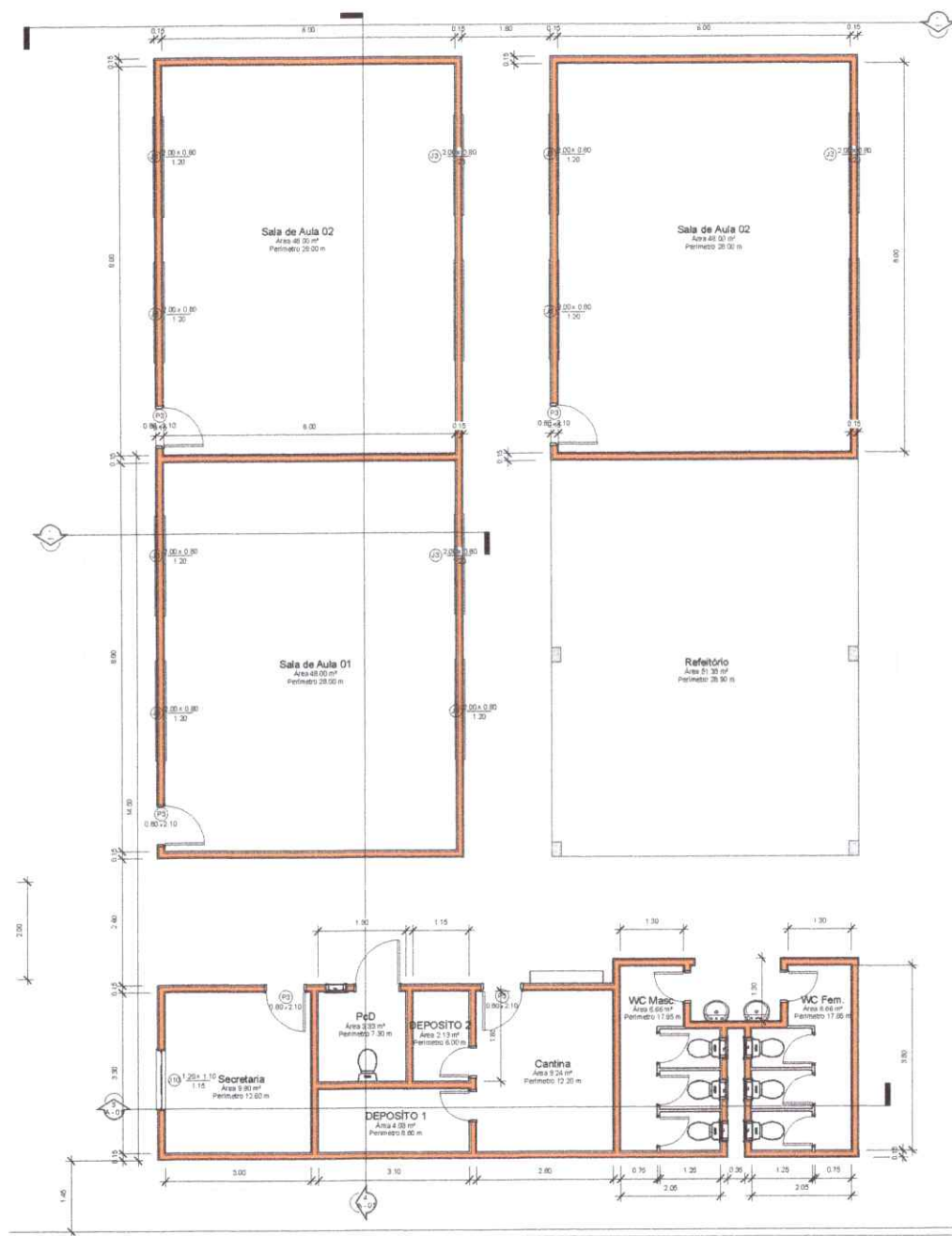
1 Planta Baixa Executiva 1:50
