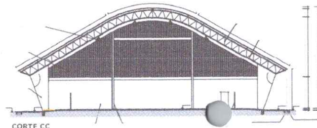
CORTE CC
