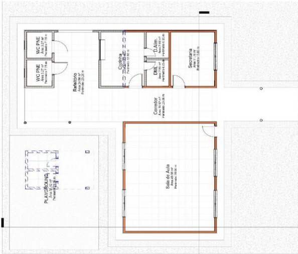
02 1:75 Planta Baixa de Demolição
