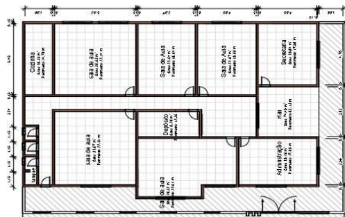
1 Planta Baixa Executiva 1 : 100
