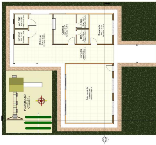
01 Planta Baixa Executiva 1:75
