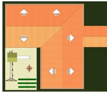
03 Estrutura do Telhado 1:125
